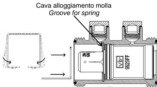
Fig.2 Inserimento molla Spring insertion
