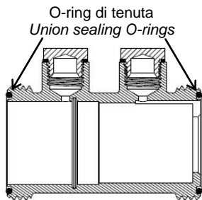
Fig.1 Corpo valvola vuoto Empty Housing
